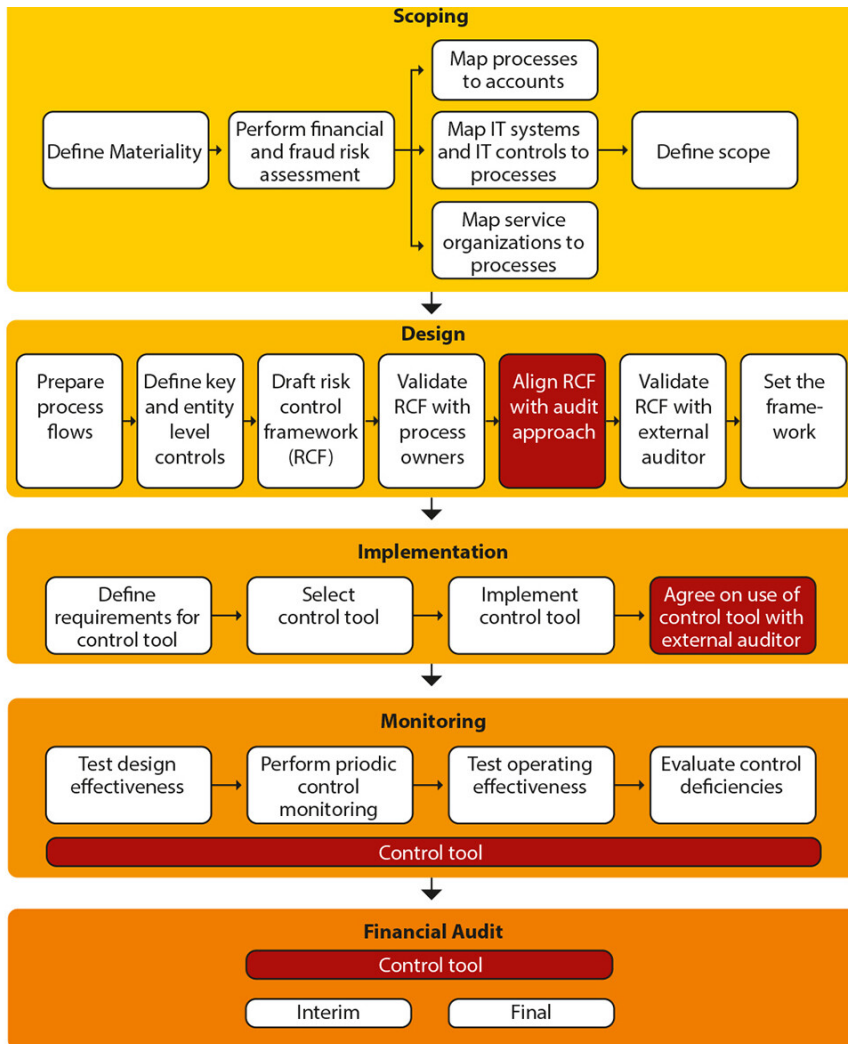
Figuur 1. Schematisch overzicht projectaanpak integrated FRCF
